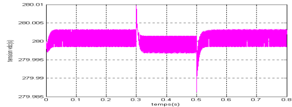
Fig. 7. DC voltage
