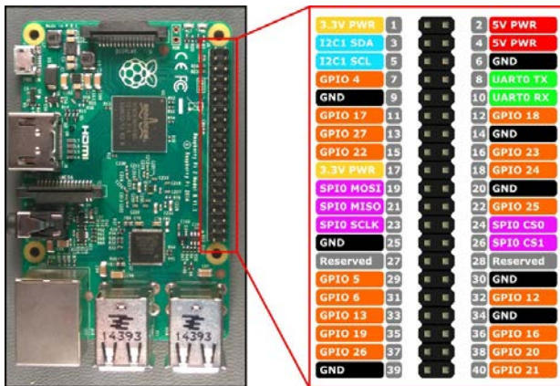
Fig. 4. GPIO [25]
